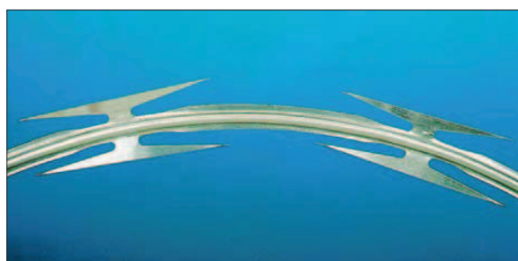
profil Rippers – w 1999 r. wdrożono do produkcji drut ostrzowy o nowym ulepszonym profilu. Zapewnia on większą sztywność i jest trudniejszy do przecięcia
